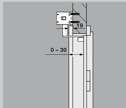
Profondità imbotte 0 – 30 mm
