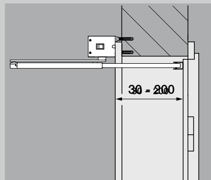
Profondità imbotte 30 – 200 mm
